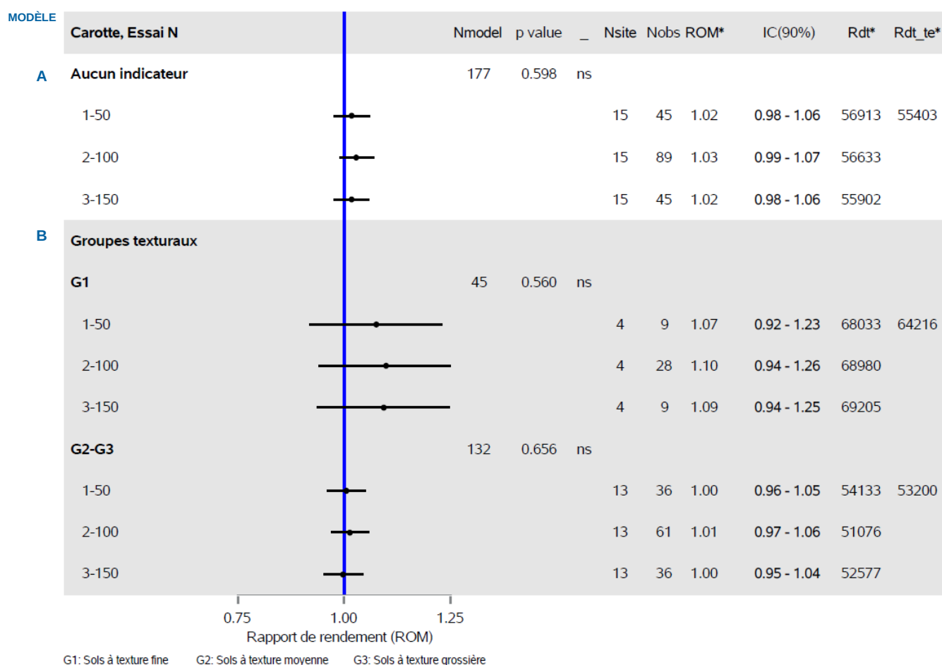
Figure 4. Résultats des analyses de variance sur la réponse de la culture aux doses croissantes d'azote. G1 : sols à texture fine ; G2 : sols à texture moyenne ; G3 : sols à texture grossière ; Nmodel : nombre d'observations du modèle ; Nsite : nombre de sites ; Nobs : nombre d'observations ; ROM : rapport de rendement (rendement parcelle fertilisée/rendement parcelle témoin) ; IC : Intervalle de confiance ; Rdt : rendement moyen en kg/ha ; Rdt_te : rendement moyen commercialisable du témoin en kg/ha ; * : Le ROM est une moyenne ajustée au modèle d'analyse de variance, tandis que le Rdt/Rdt_te est une moyenne arithmétique. De ce fait, le rapport entre le Rdt et le Rdt_te peut ne pas donner la valeur exacte du ROM.
