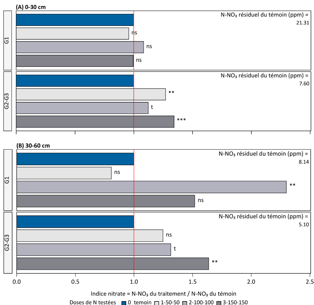
Figure 6. Nitrate résiduel (N-NO 3 ) à la récolte dans les couches de sol 0-30 cm (A) et 30-60 cm (B) en fonction des doses d'azote et des groupes de textures pour la carotte. G1 : sols à texture fine ; G2 : sols à texture moyenne ; G3 : sols à texture grossière. Les statistiques ont été réalisées sur les données transformées (log), alors que le graphique présente les données brutes tels qu'analysés au laboratoire. De ce fait, les résultats du test statistique pourraient ne pas correspondre exactement aux données présentées sur le graphique. ns : non significatif ; t : tendance, P < 0,12 ; * significatif, P < 0,05 ; ** significatif, P < 0,01 .
