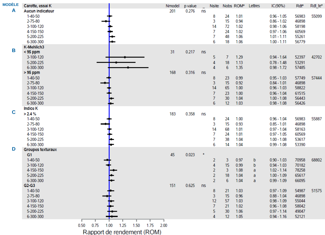
Figure 9. Résultats des analyses de variance sur la réponse de la culture aux doses croissantes de potassium. Nmodel : nombre d'observations du modèle ; Nsite : nombre de sites ; Nobs : nombre d'observation ; ROM : rapport de rendement (rendement parcelle fertilisée/rendement parcelle témoin) ; G1 : sols à texture fine ; G2 : sols à texture moyenne ; G3 : sols à texture grossière ; IC : intervalle de confiance ; Rdt = rendement moyen commercialisable (kg/ha) ; rdt_te = rendement moyen commercialisable du témoin (kg/ha) ; * : Le ROM est une moyenne ajustée au modèle d'analyse de variance, tandis que le Rdt/Rdt_te est une moyenne arithmétique. De ce fait, le rapport entre le Rdt et le Rdt_te présentés ci-dessus peut ne pas donner la valeur exacte du ROM.
