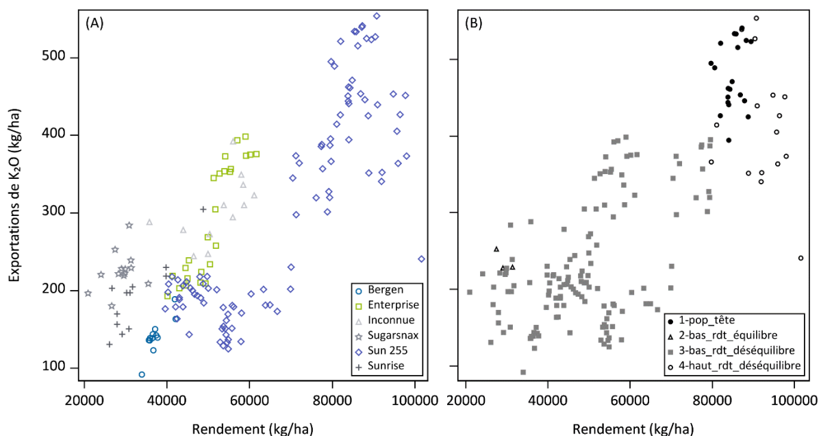
Figure 10. Exportations de potassium en fonction des rendements de la carotte, exprimés selon les variétés (A) et selon le diagnostic nutritionnel (B).
