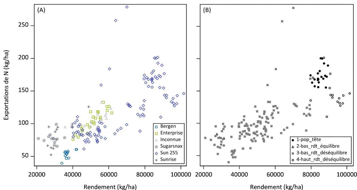
Figure 5. Exportations d'azote en fonction des rendements de la carotte, exprimés selon les variétés (A) et selon le diagnostic nutritionnel (B).
