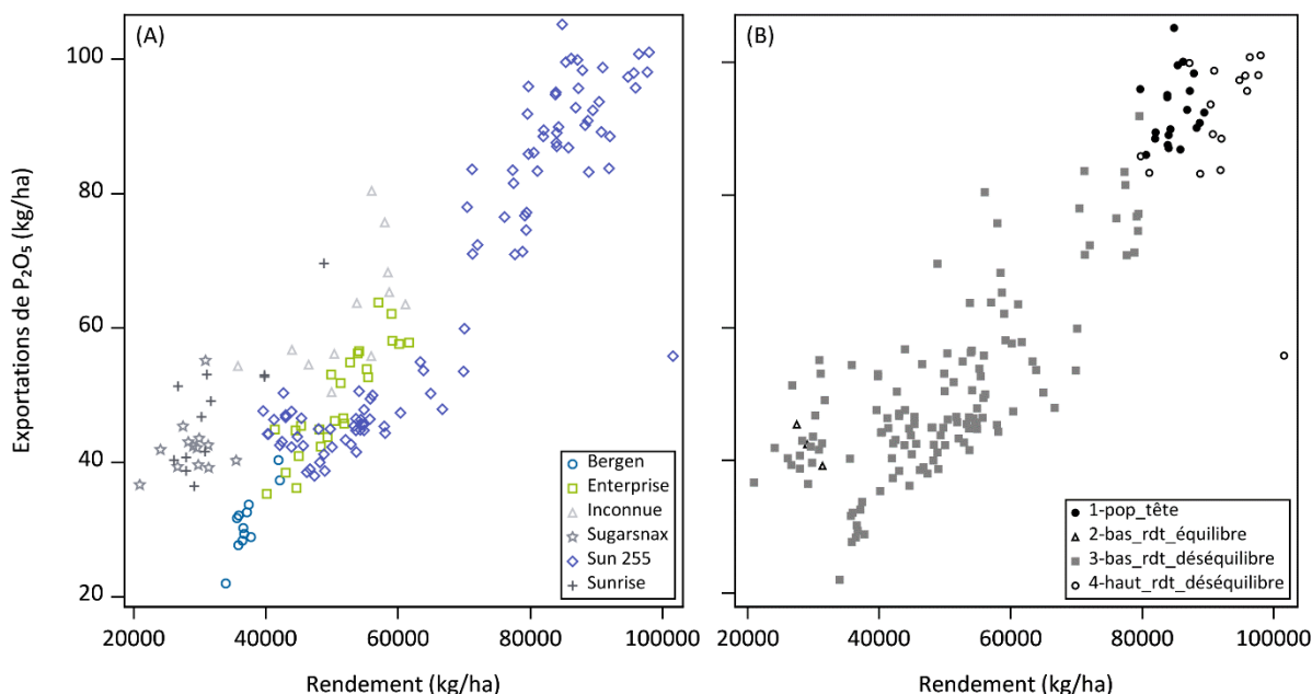
Figure 8. Exportations de phosphore en fonction des rendements de la carotte, exprimés selon les variétés (A) et selon le diagnostic nutritionnel (B).
