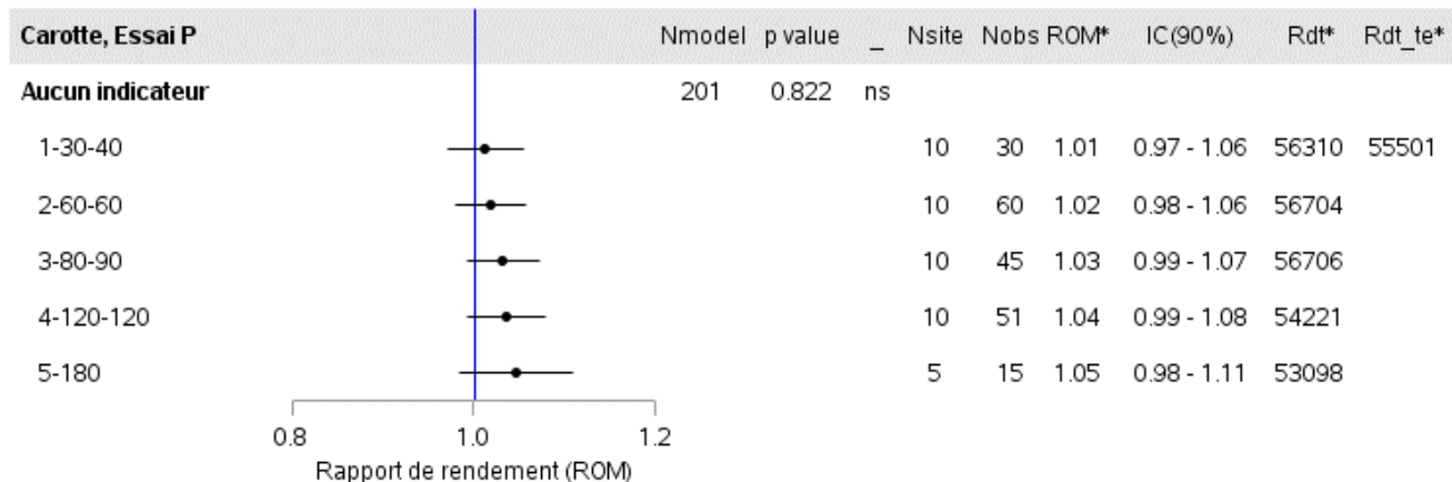
Figure 7. Résultats des analyses de variance sur la réponse de la culture aux doses croissantes de phosphore. Nmodel : nombre d'observations du modèle ; Nsite : nombre de sites ; Nobs : nombre d'observation ; ROM : rapport de rendement (ROM = rendement parcelle fertilisé/rendement parcelle témoin) ; IC : Intervalle de confiance ; Rdt : rendement moyen en kg/ha ; Rdt_te : rendement moyen commercialisable du témoin en kg/ha ; * : Le ROM est une moyenne ajustée au modèle d'analyse de variance, tandis que le Rdt/Rdt_te est une moyenne arithmétique. De ce fait, le rapport entre le Rdt et le Rdt_te présentés ci-dessus peut ne pas donner la valeur exacte du ROM.
